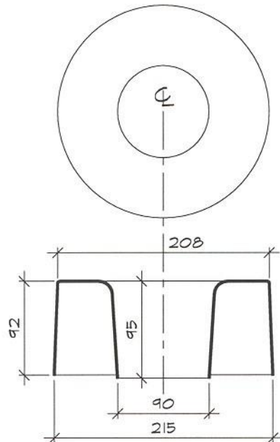
Capuchon modèle 1824
