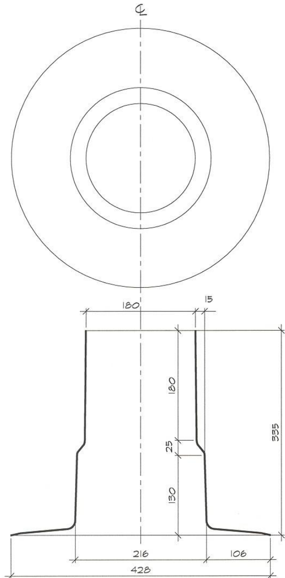
Manchon d'évent, modèle 1700
