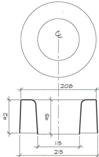
Capuchon modèle 1825
