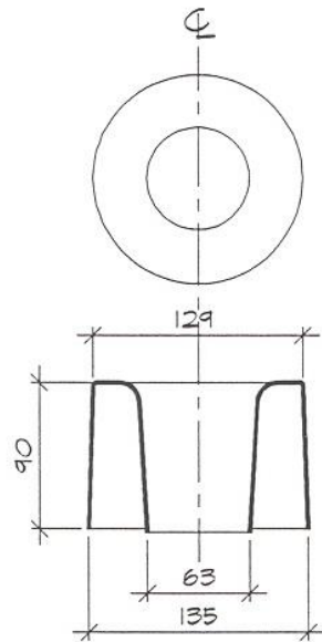
Capuchon, modèle 1523
