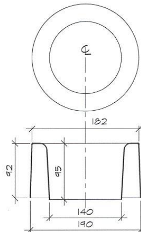
Capuchon. modèle 1726
