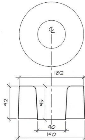
Capuchon. modèle 1724
