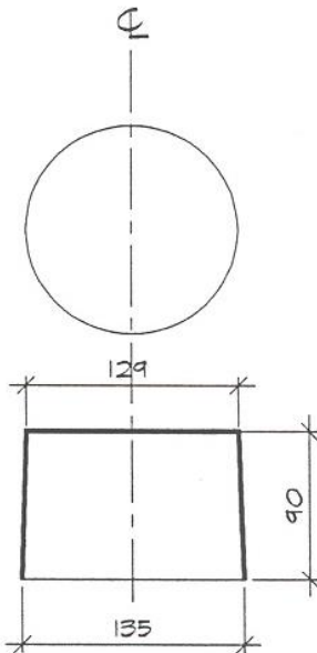
Capuchon, modèle 1505
