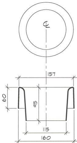
Capuchon. modèle 1625
