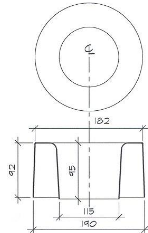
Capuchon. modèle 1725
